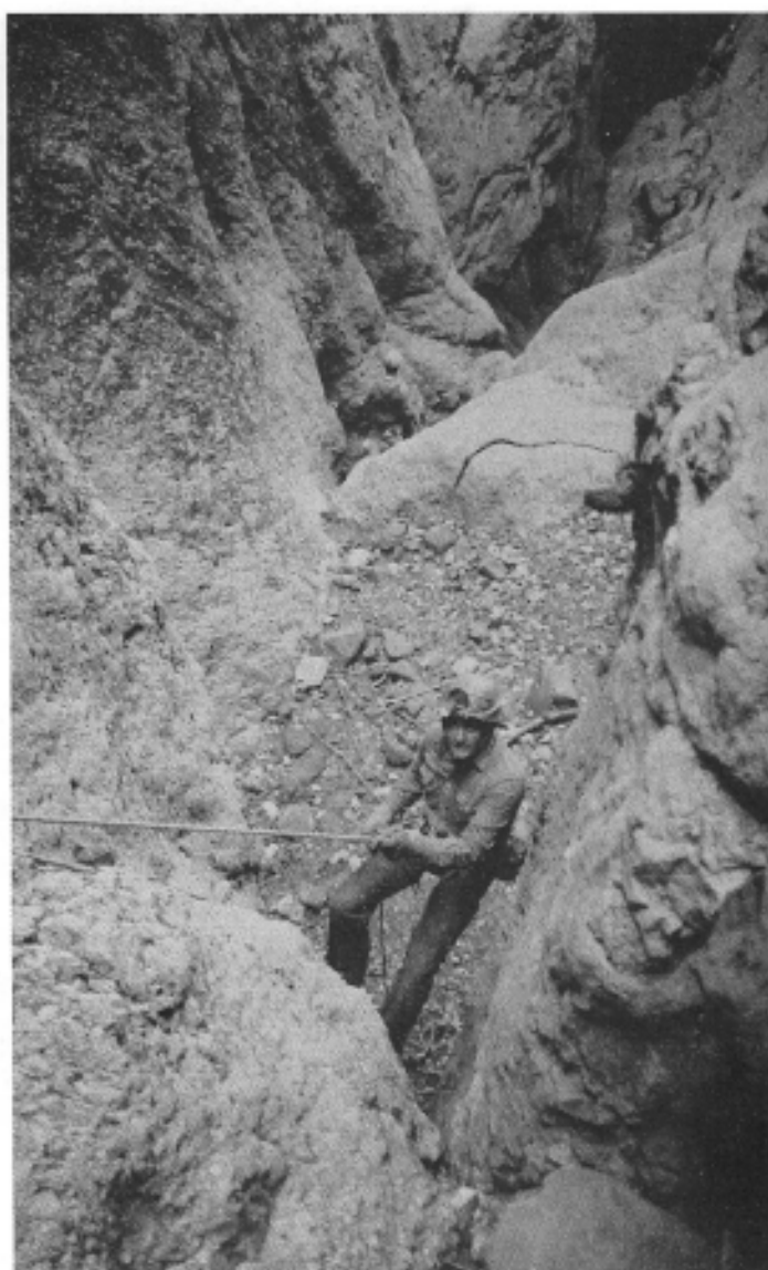
Photos 32: Succession de ressauts et de marmites qui longent la faille.
