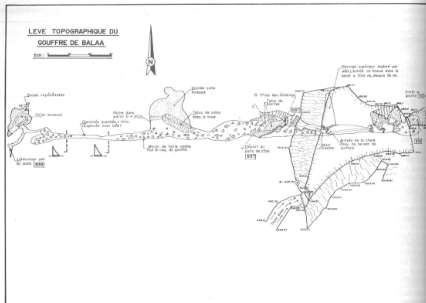
Figure 18: Plan et coupe du gouffre de Balaa (18a et 18b).
